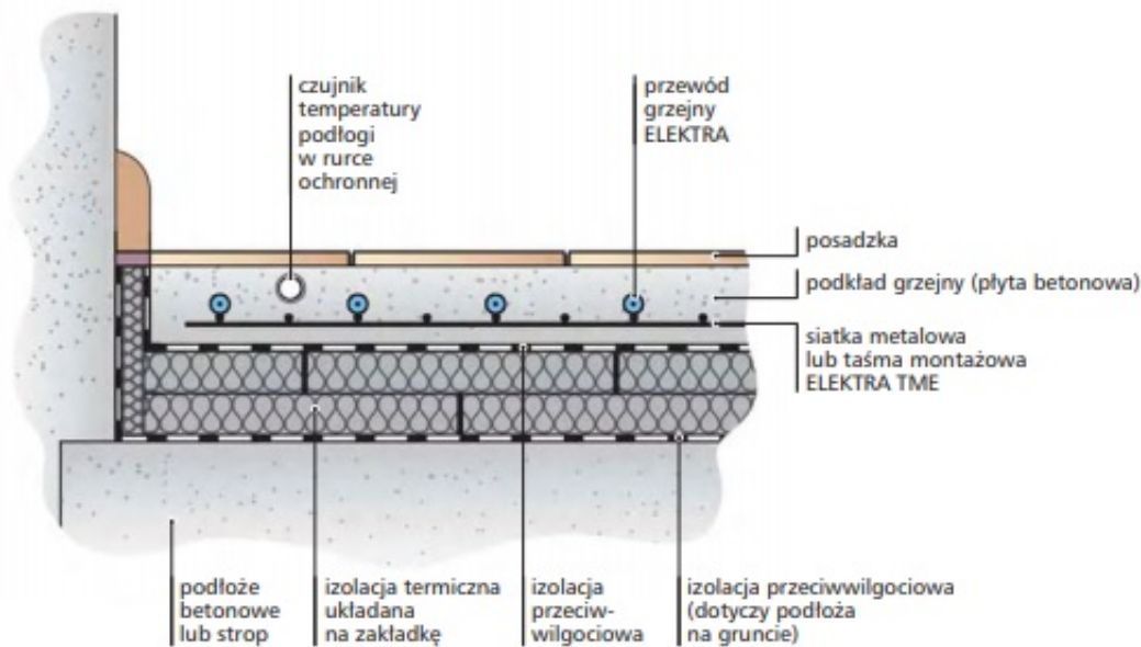
Przekrój podłogi
