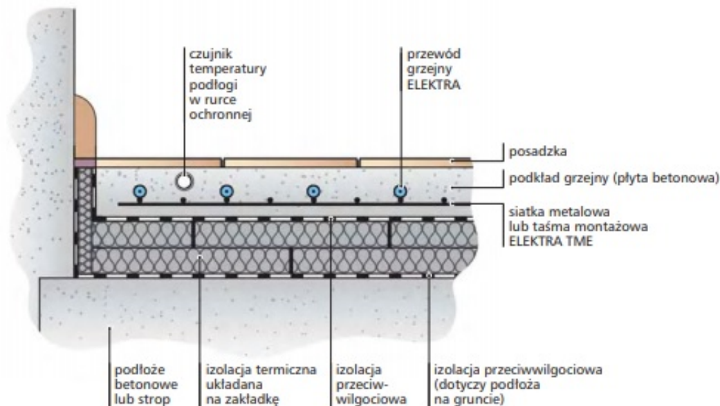
Przekrój podłogi
