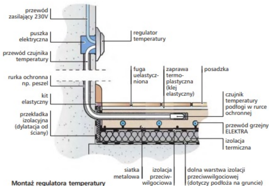
Montaż regulatora temperatury
